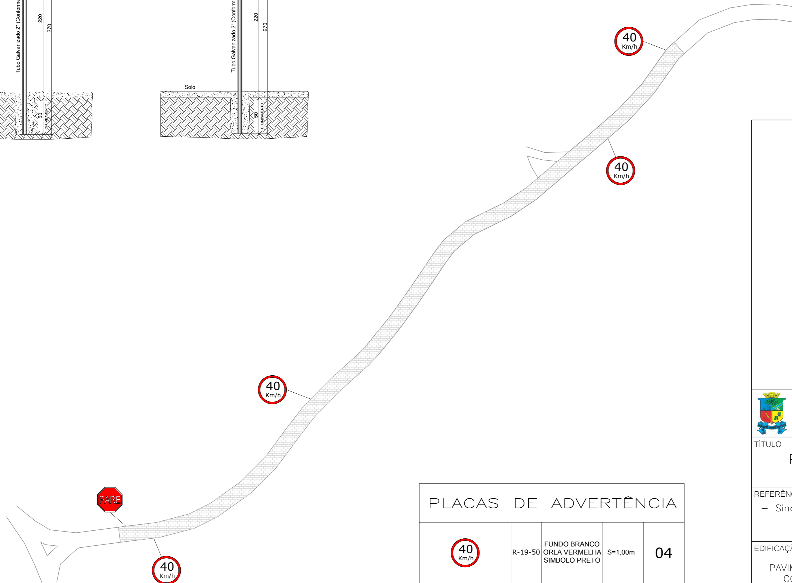
PLANTA DE SINALIZAÇÃO
