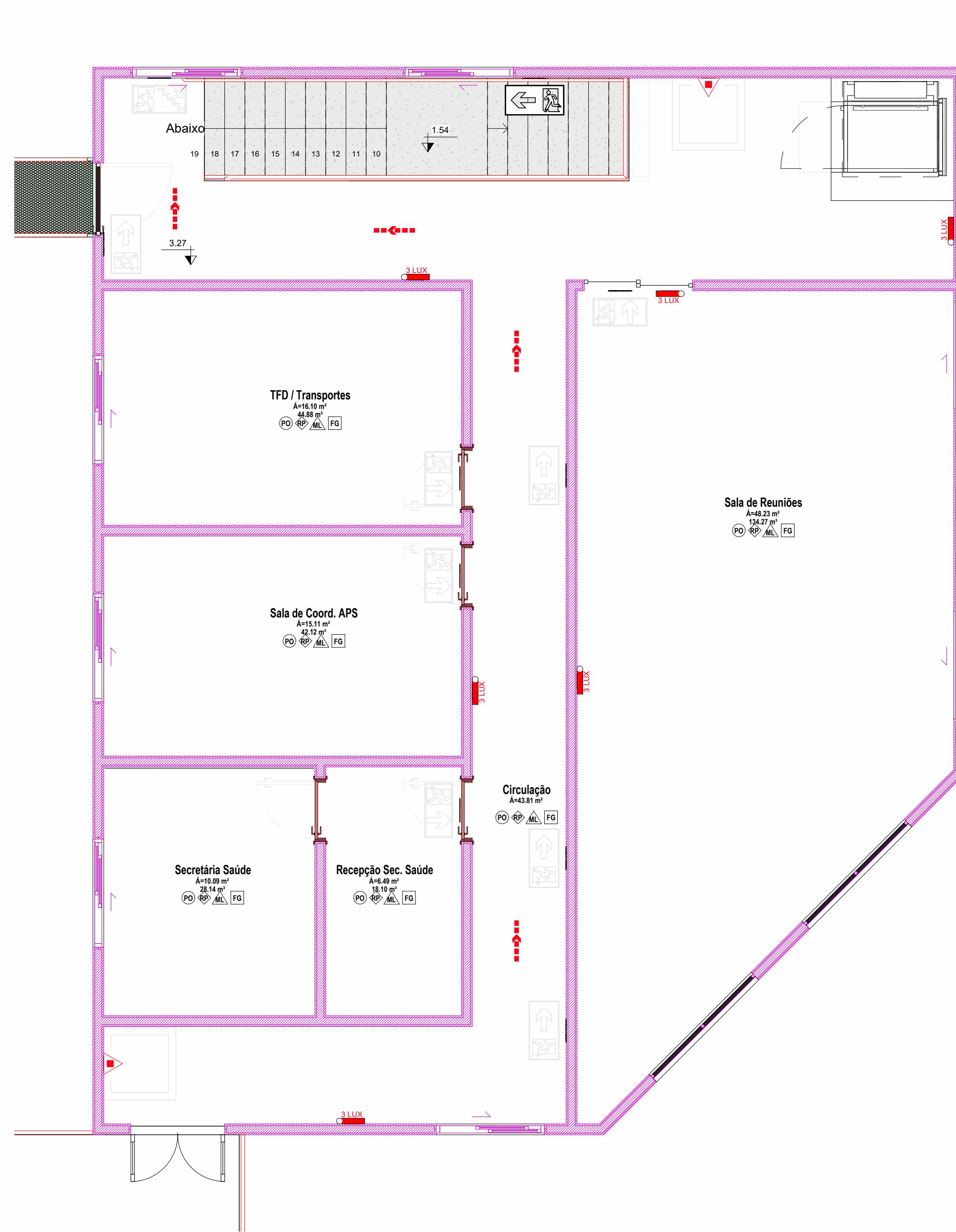
2 1º piso ESCALA: 1 : 50
