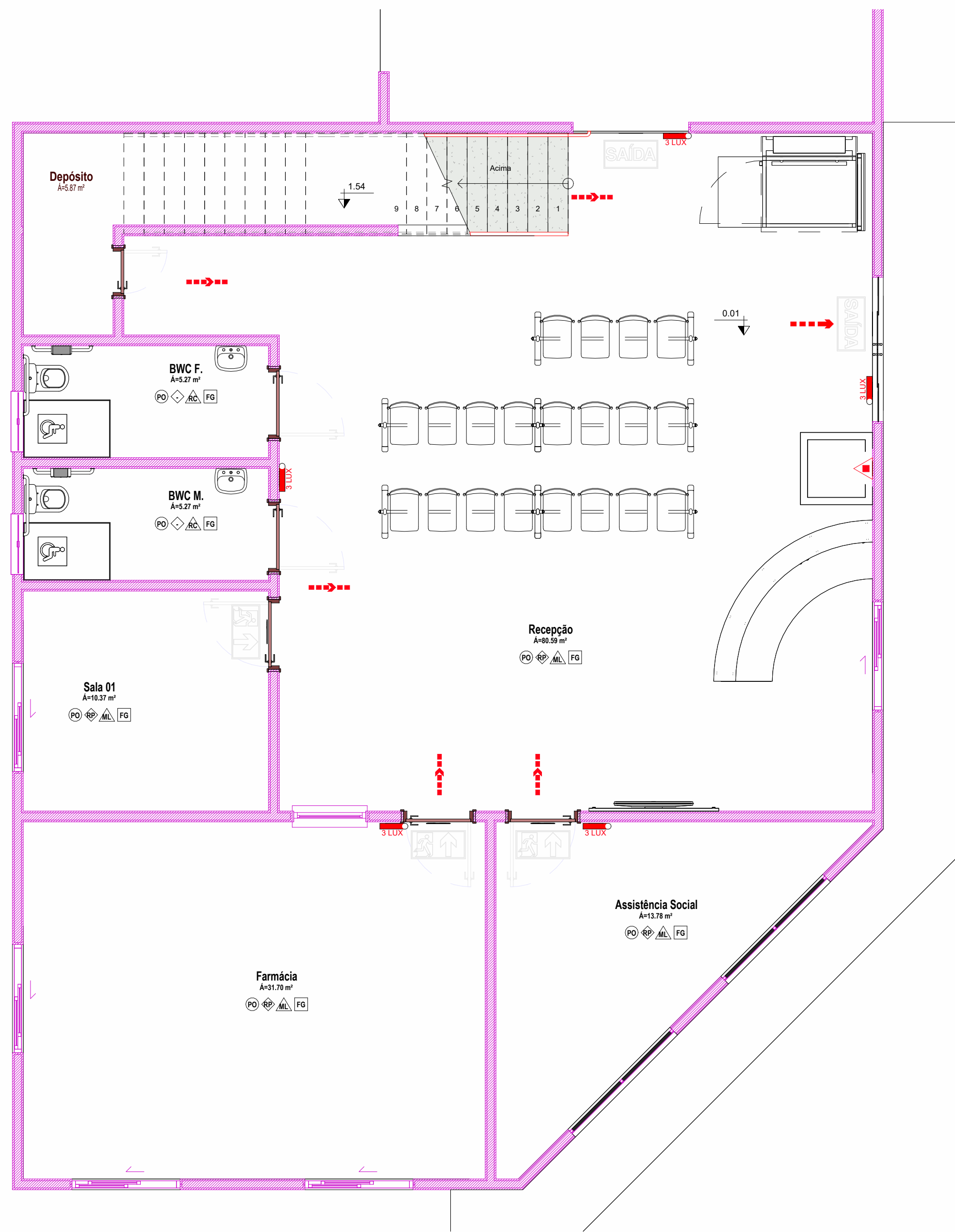
1 Piso térreo ESCALA: 1 : 50
