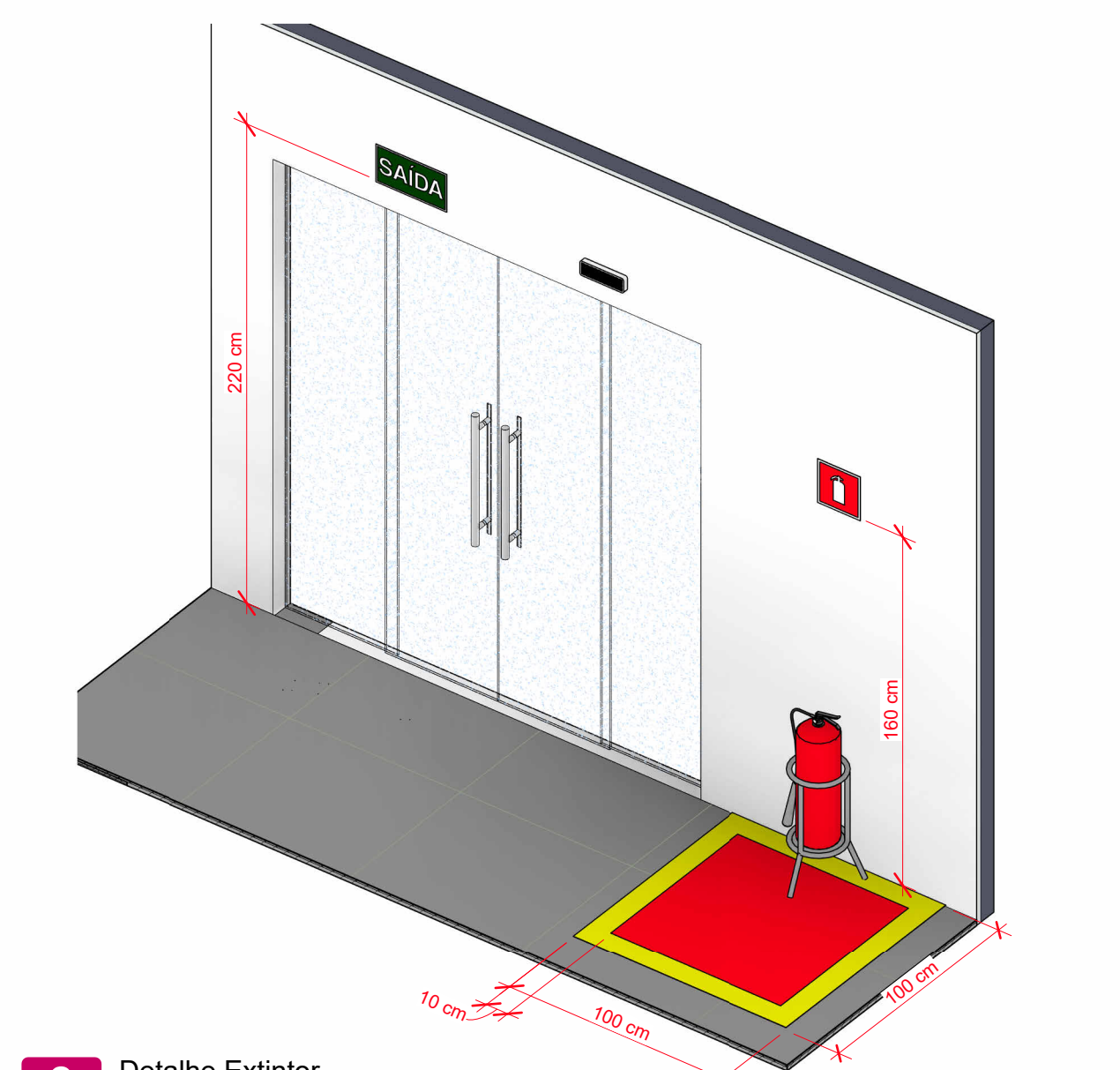
3 Detalhe Extintor ESCALA:
