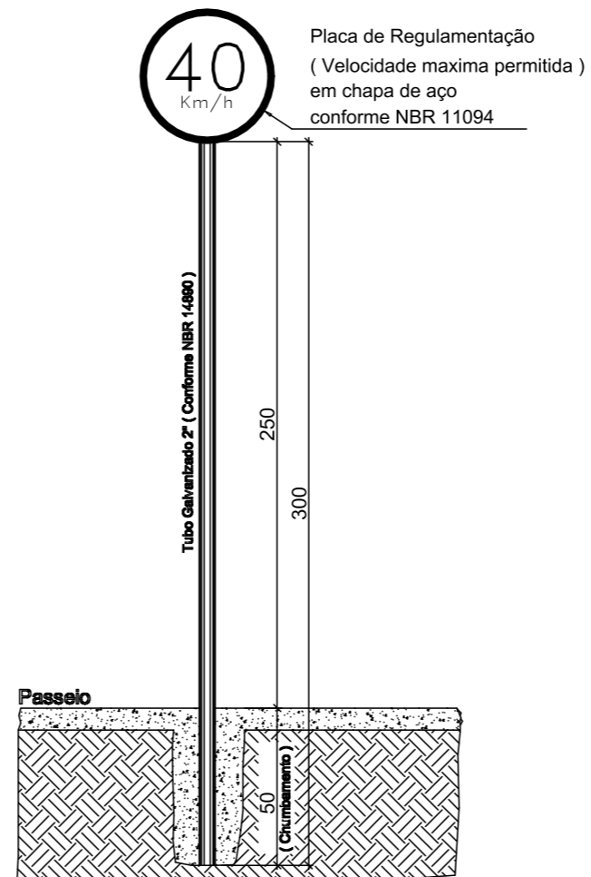
DETALHE ESQUEMATICO ESC: 1/15 CONFORME NBR 14962
