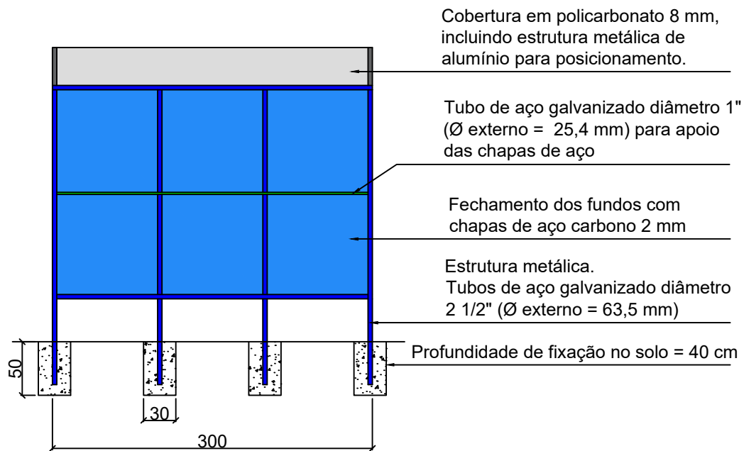
CORTE 1 - FUNDOS
