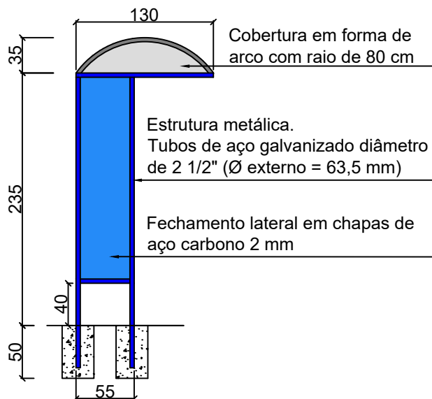
CORTE 2 - LATERAL
