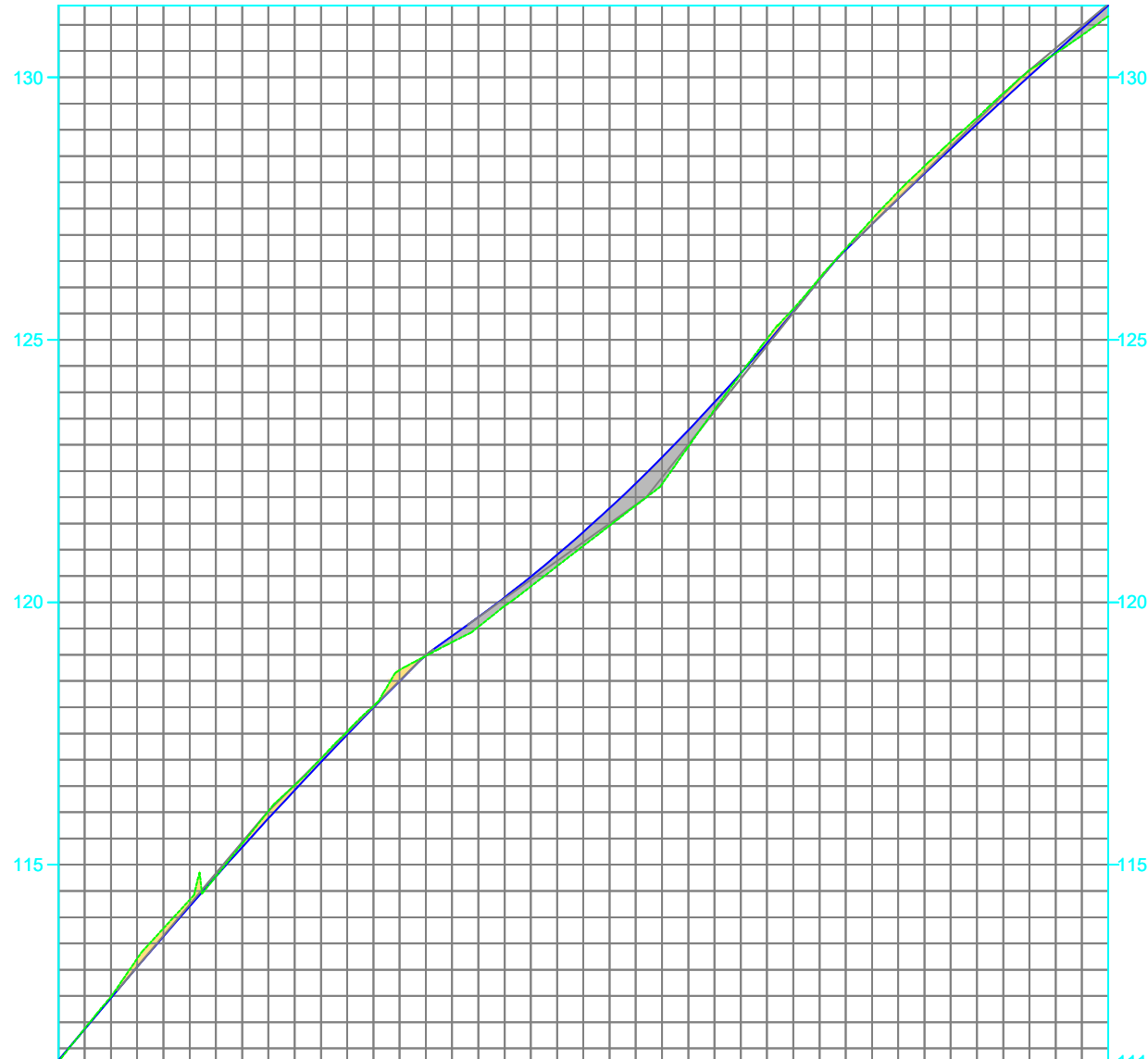
PERFIL LINHA UNIÃO
