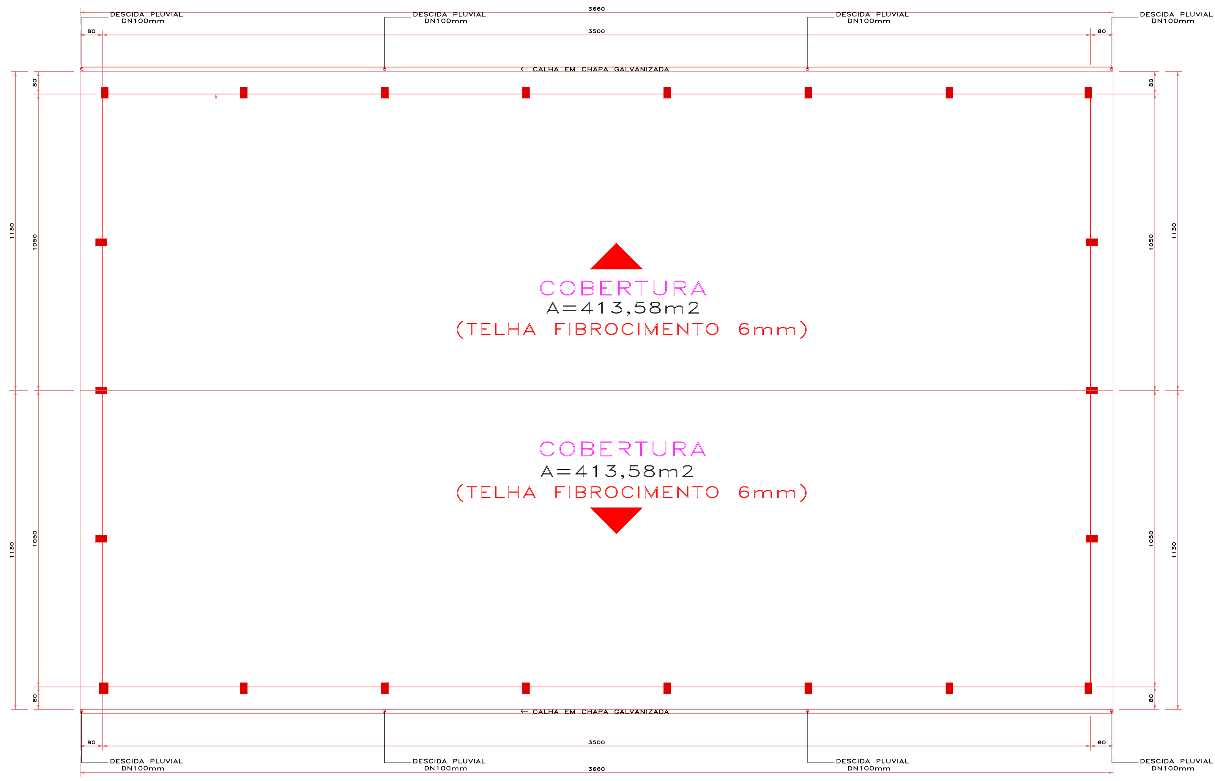
PLANTA DE COBERTURA CAPTAÇÃO ÁGUAS PLUVIAIS ESC. 1 / 75
