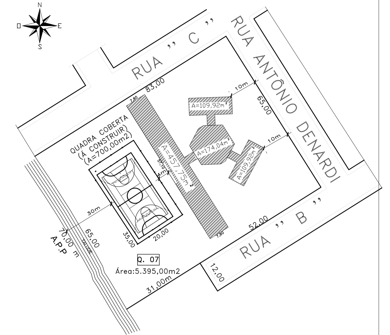
SITUAÇÃO GENÉRICA ESC. 1/125
