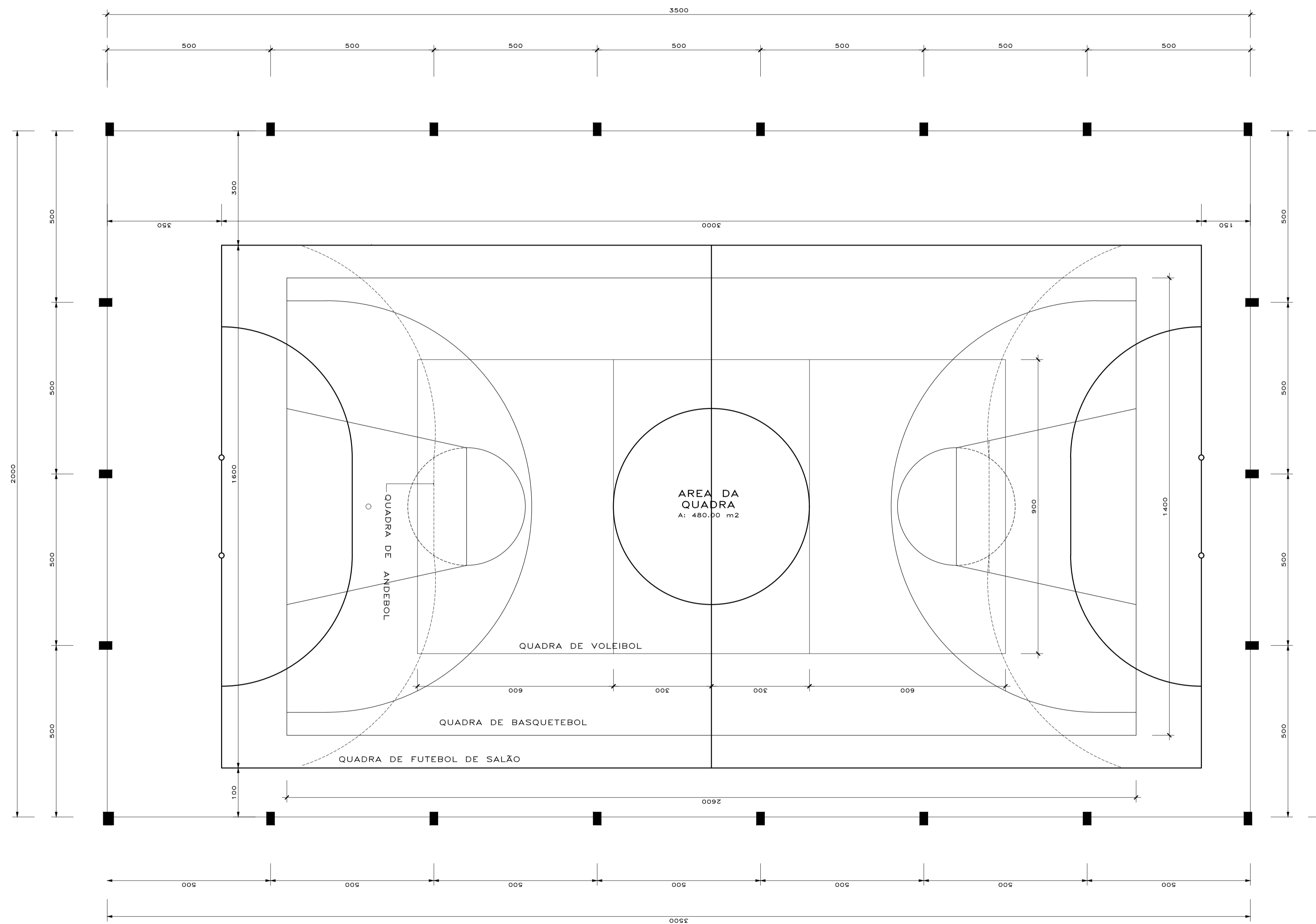
PLANTA BAIXA ESC. 1 / 75 ÁREA = 700,00m 2
