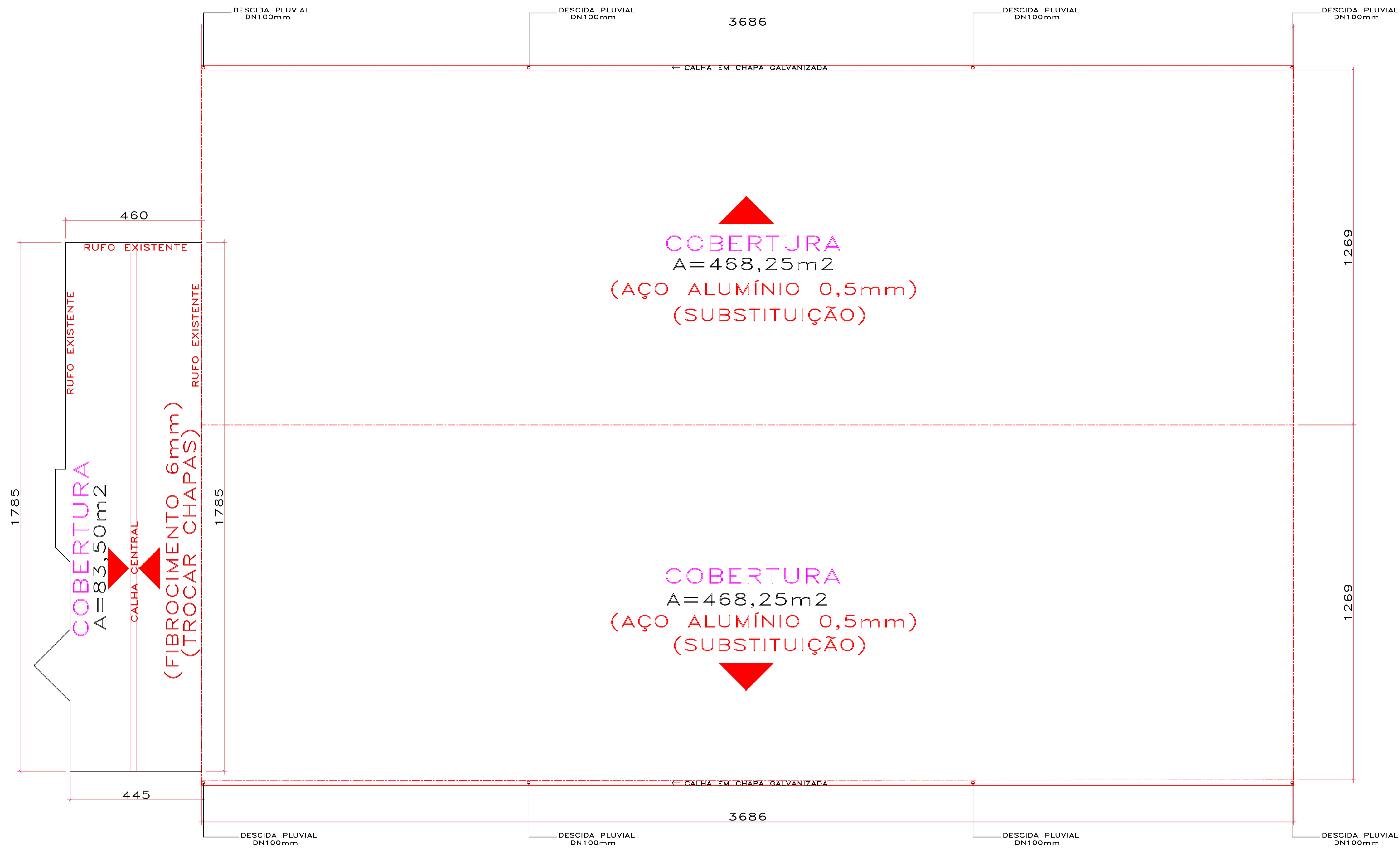
PLANTA DE COBERTURA CAPTAÇÃO ÁGUAS PLUVIAIS ESC. 1 / 75
