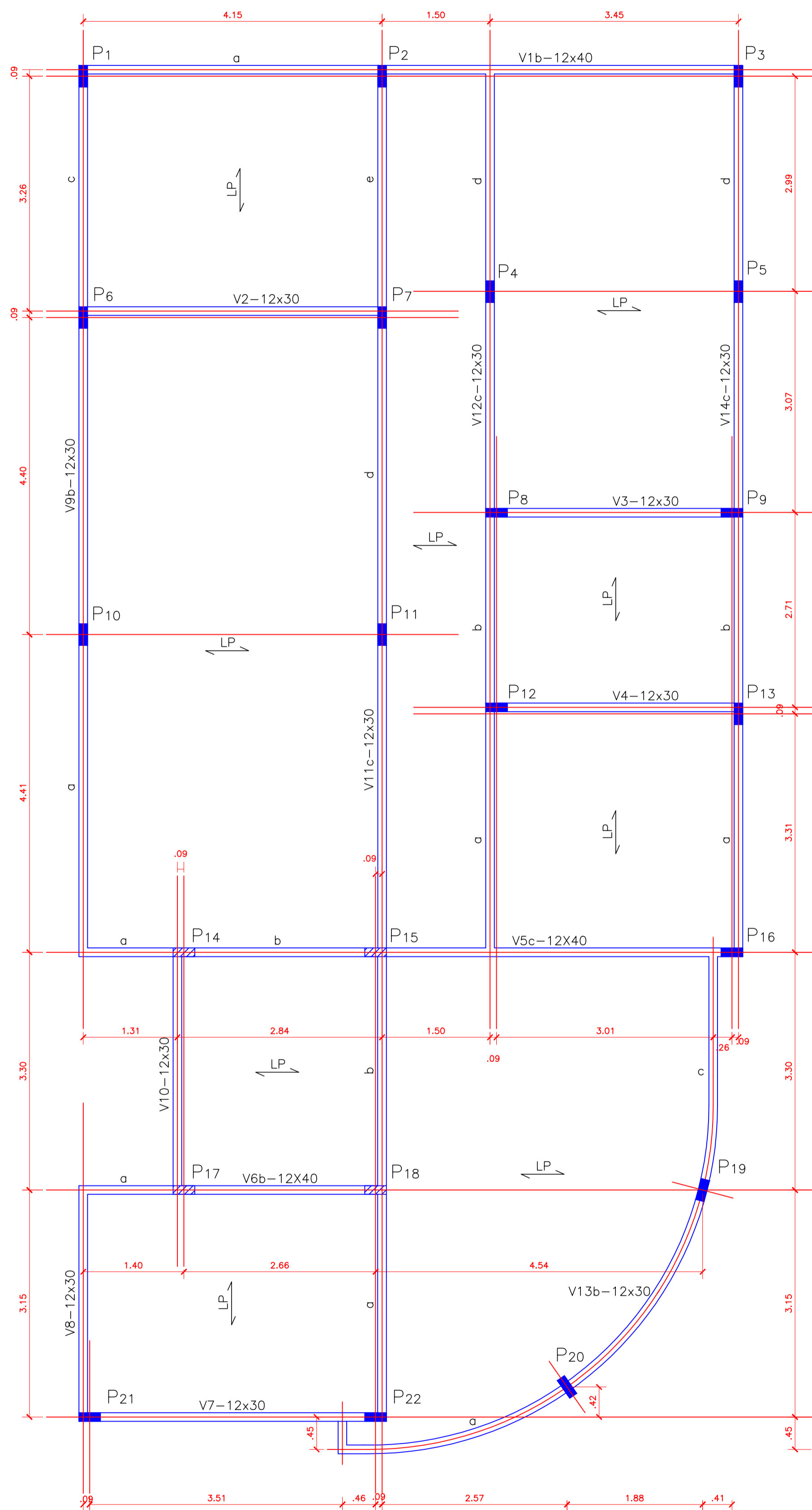
CRAS FORMA DE VIGAS
