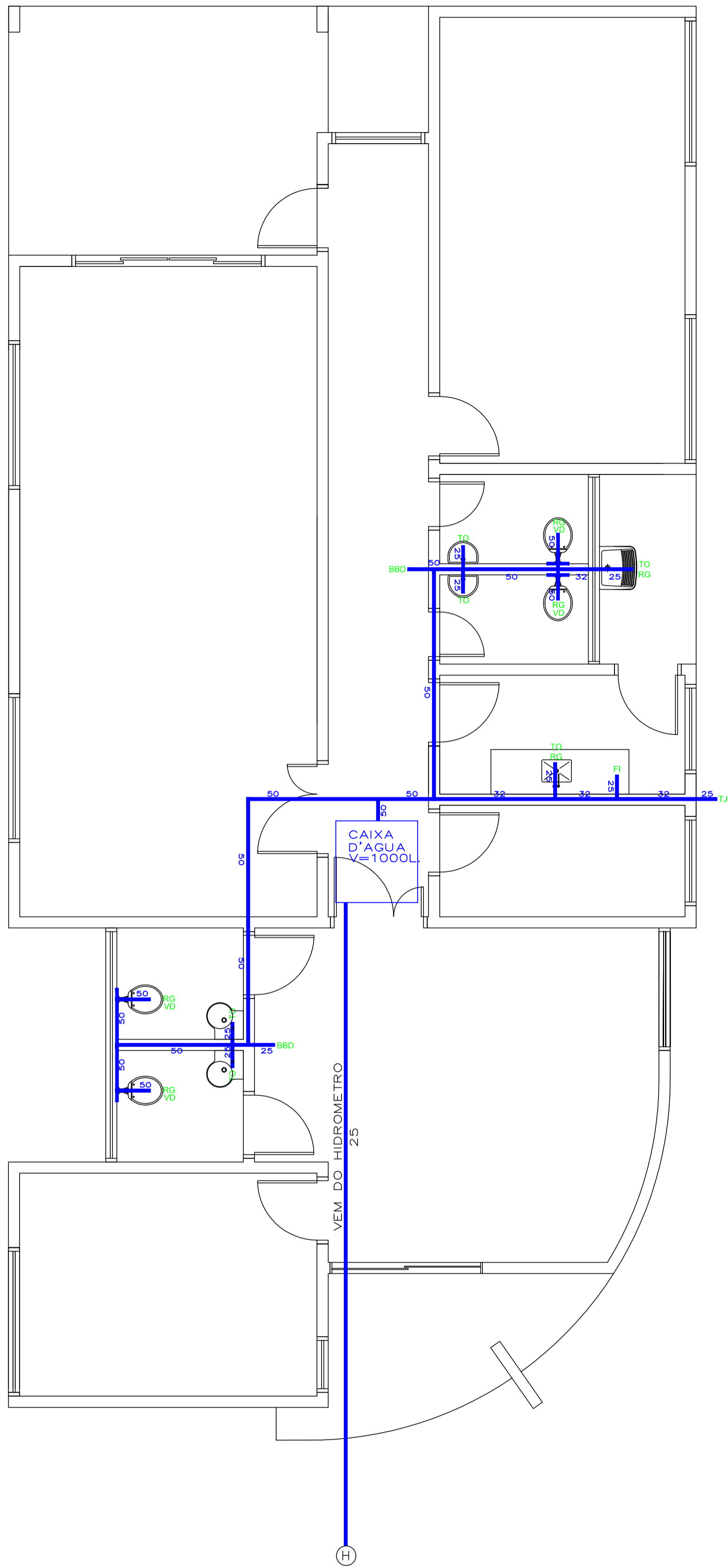
CRAS – PROJETO HIDRÁULICO
