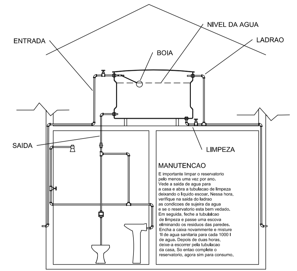
DETALHE CAIXA D'AGUA
