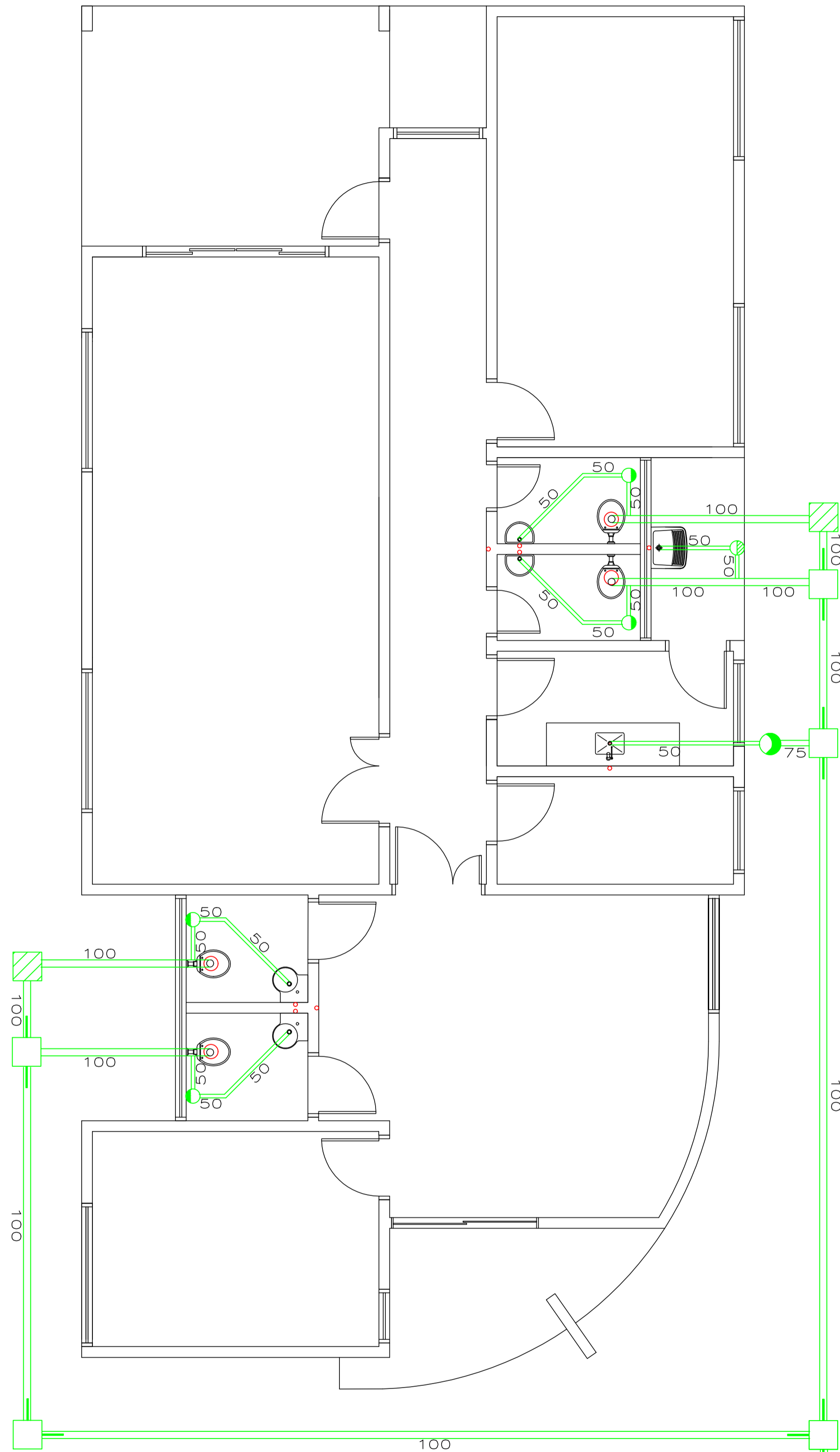
CRAS – PROJETO SANITÁRIO
